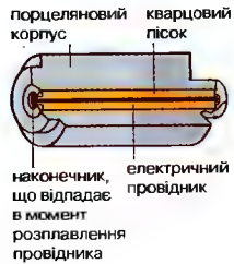
Запобіжник електричний плавкий Протікання надмірного струму спричинює плавлення провідника в середині запобіжника і розрив електричного кола
